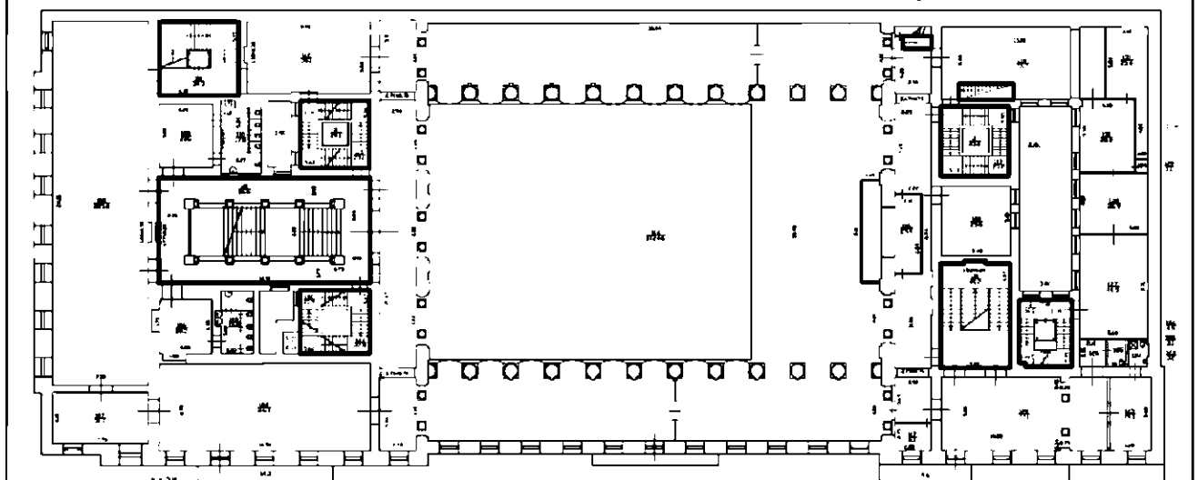
Схема лестниц на плане 2-го этажа
