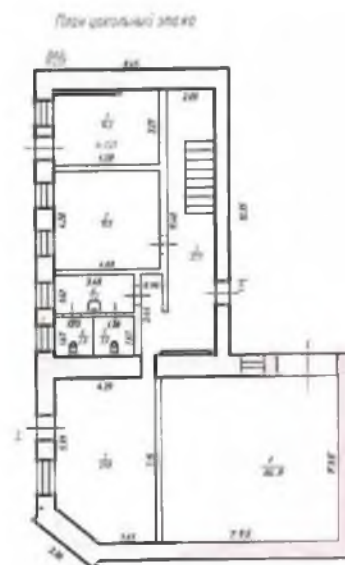
План цокольного этажа
