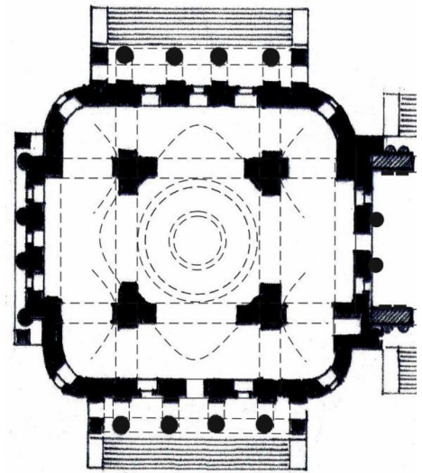
План-схема основного объёма
