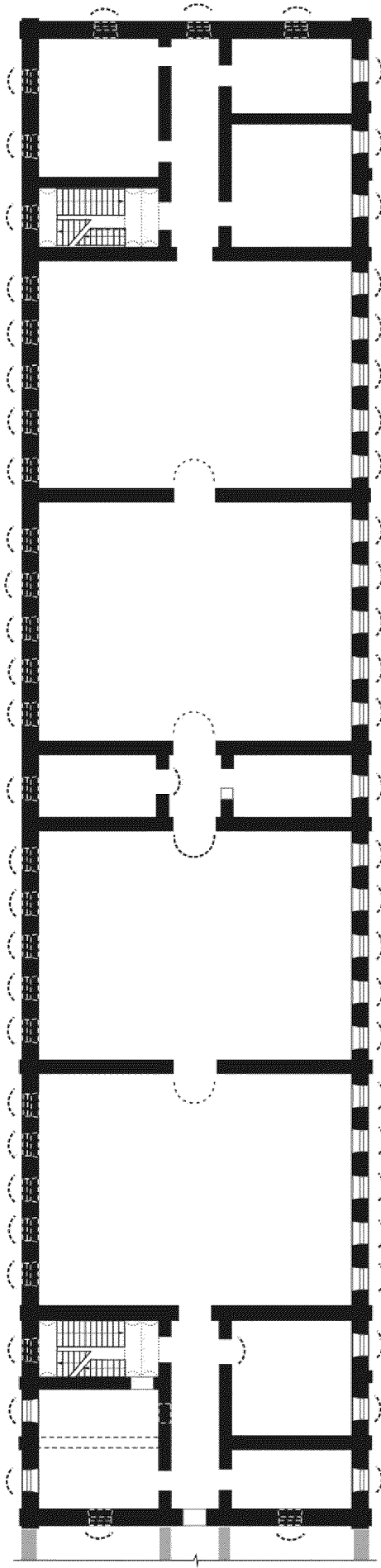
План 2 этажа
