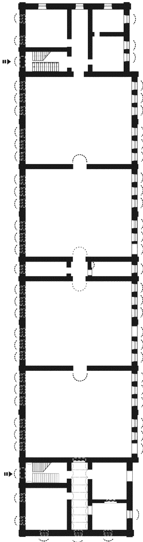
План 1 этажа
