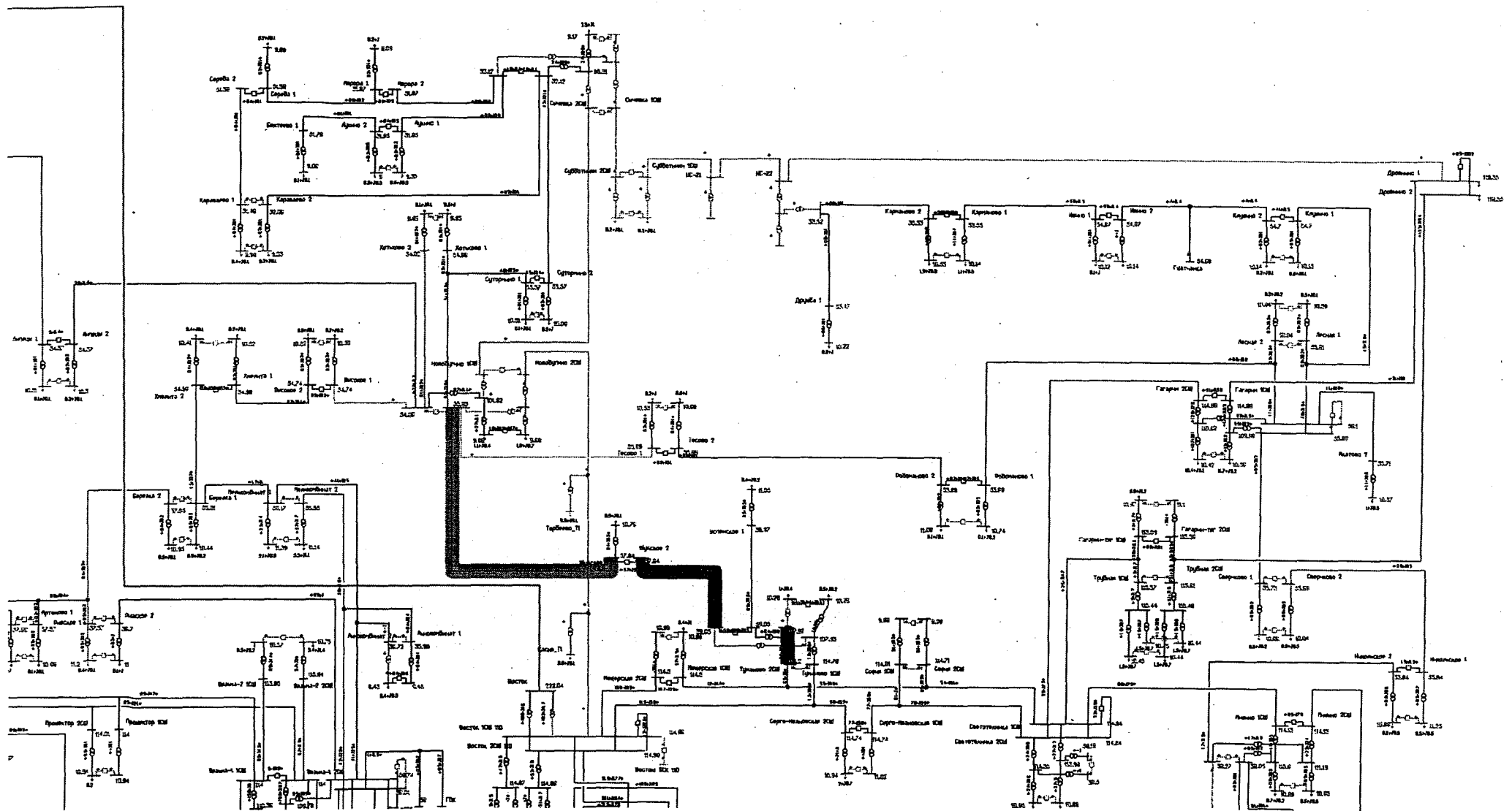
Рис. 2. Результат расчета режима (ограничение потребителей ПС 110 кВ Сычевка)
