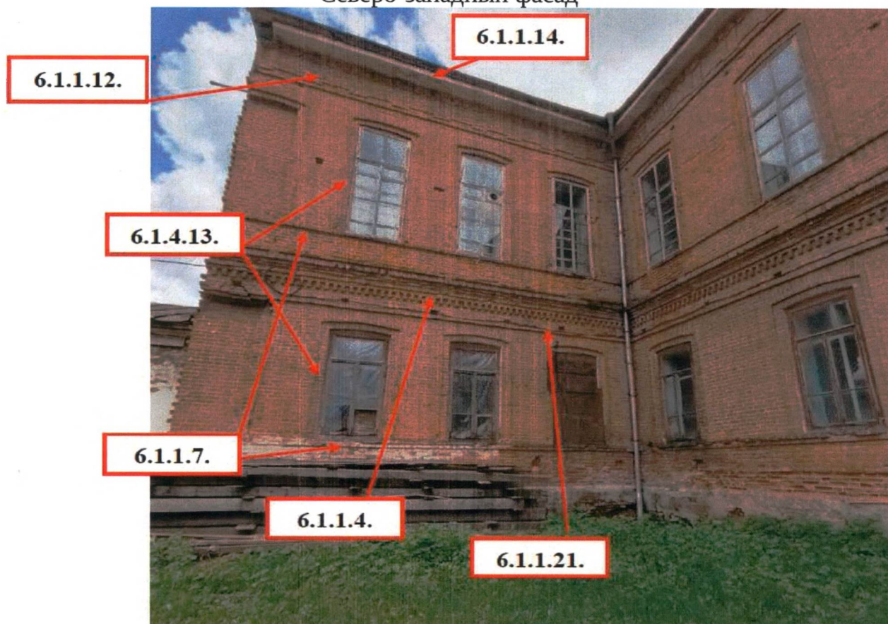
Северо-западный фасад
