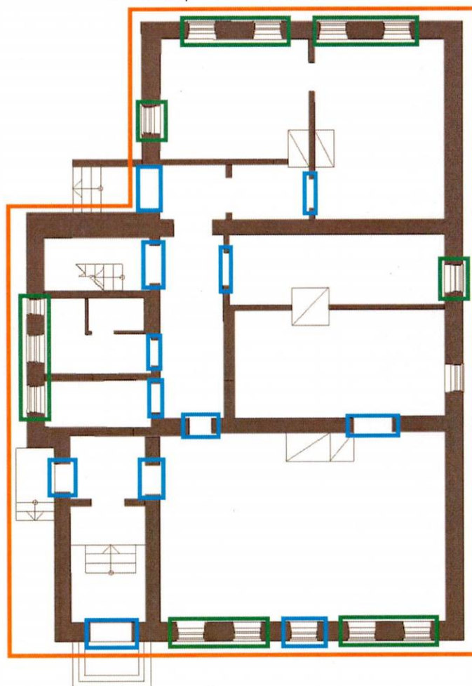
План цокольного этажа
