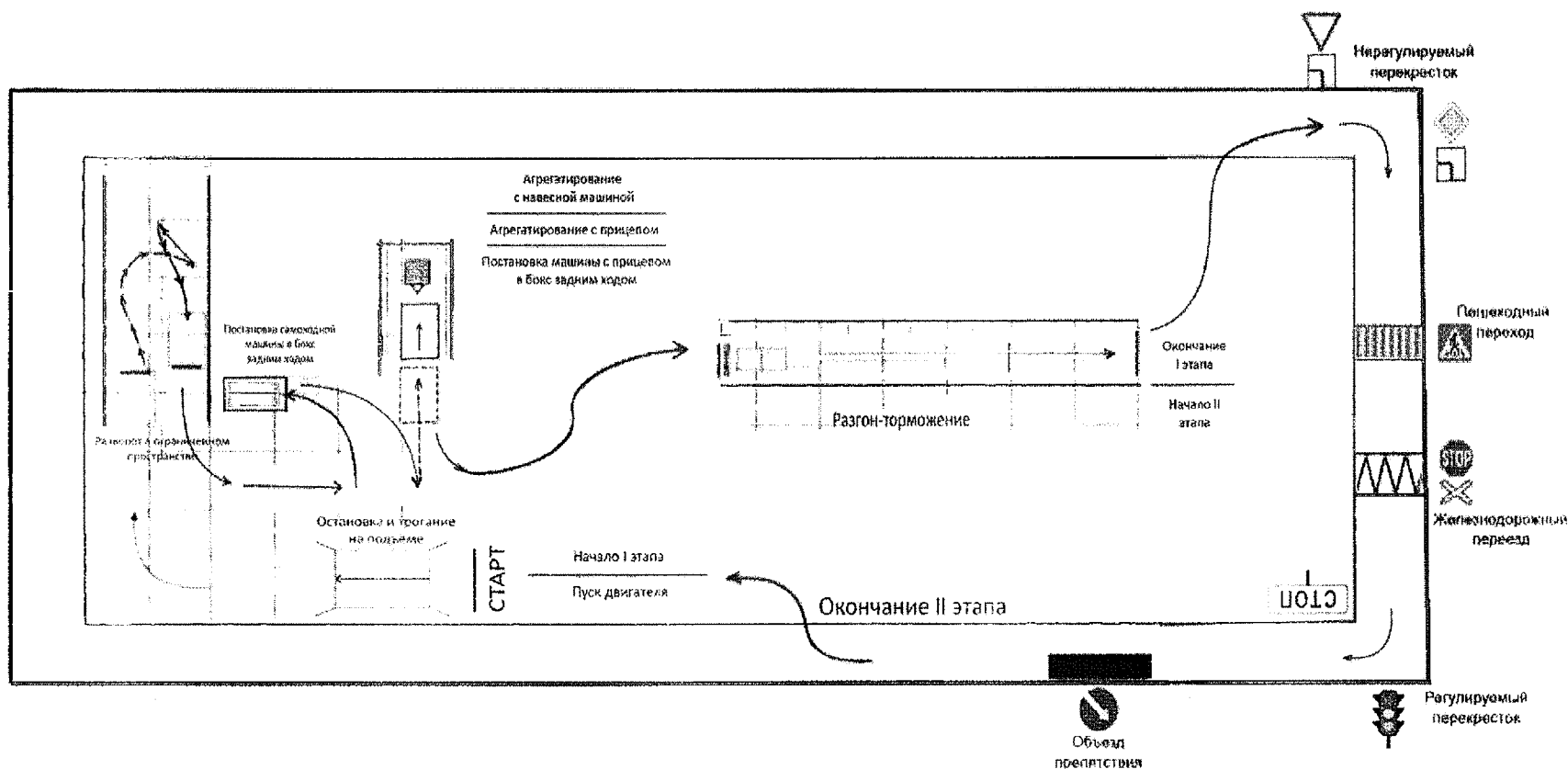
Рисунок 1. Примерная схема площадки (трактородрома) для проведения I и II этапов практического экзамена на право управления самоходными машинами
