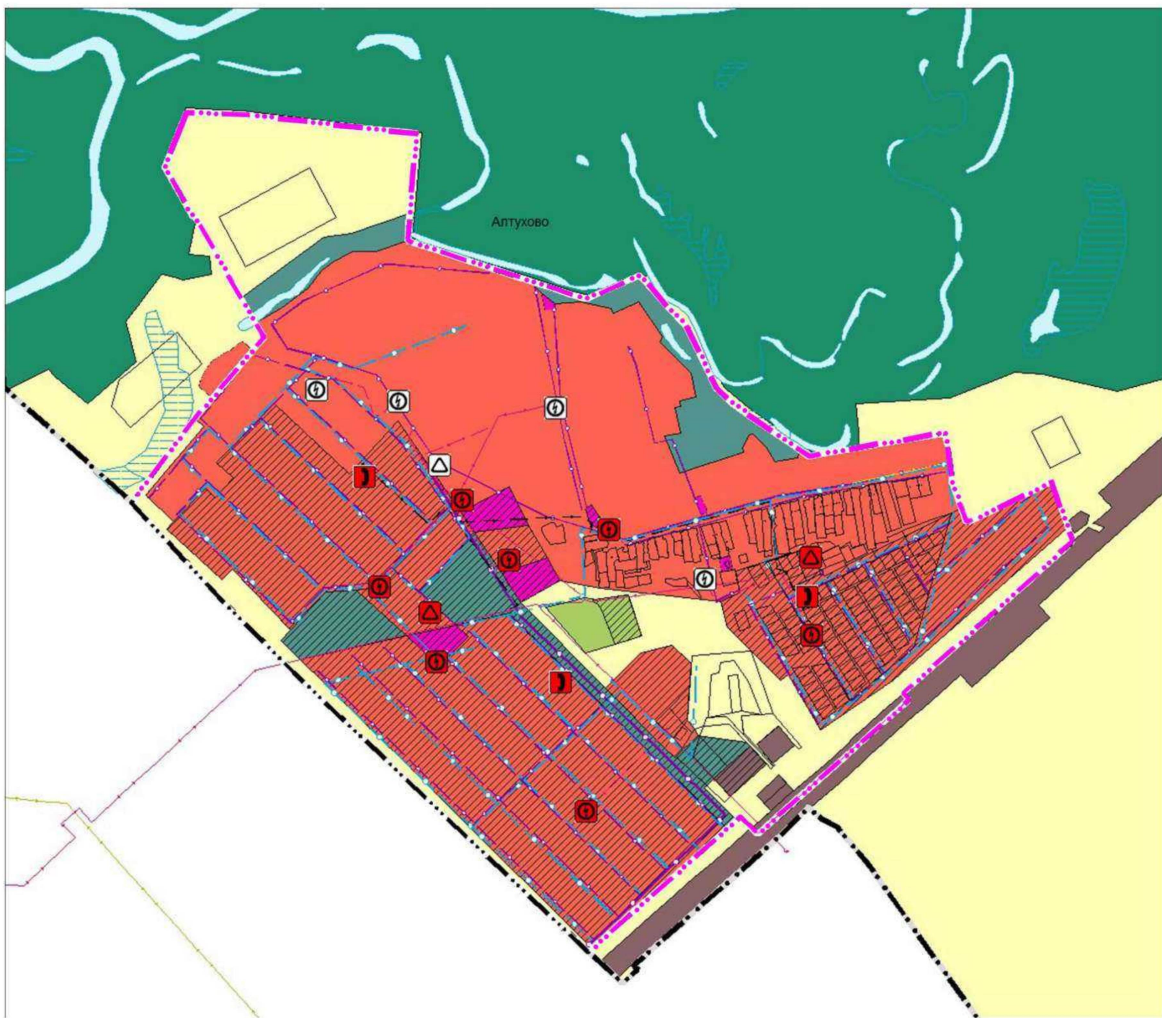
Карта планируемого размещения объектов инженерной инфраструктуры местного значения с. Свободные Ключи, п. Най-Лебен муниципального района Кинель-Черкасский Самарской области
