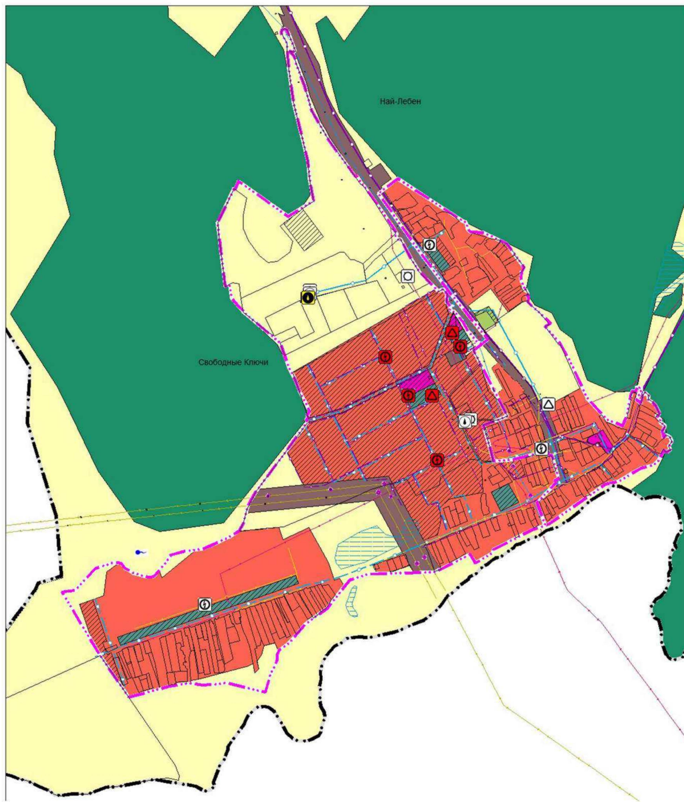
Карта планируемого размещения объектов инженерной инфраструктуры местного значения с. Свободные Ключи, п. Най-Лебен муниципального района Кинель-Черкасский Самарской области
