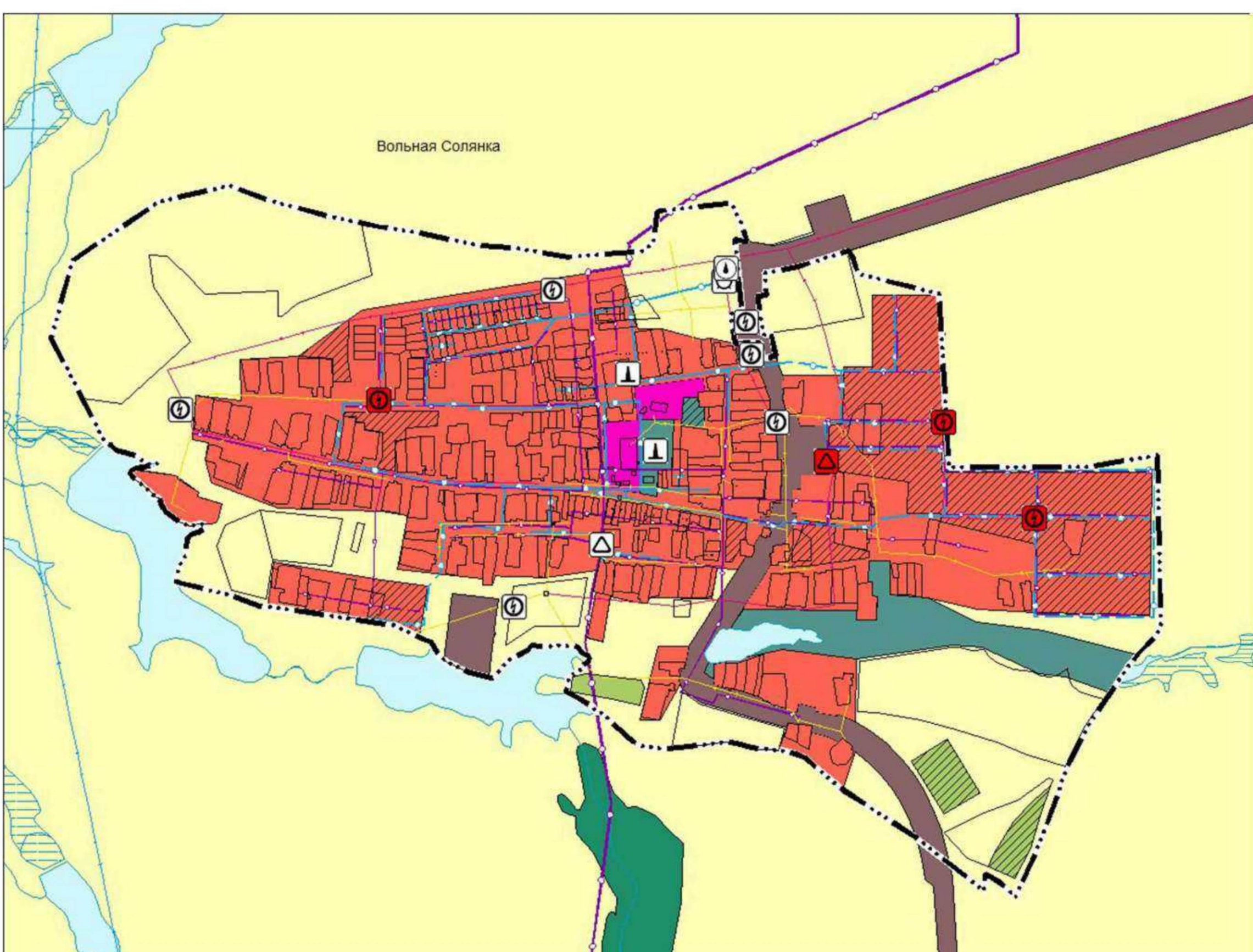
Карта планируемого размещения объектов инженерной инфраструктуры местного значения с. Алтухово муниципального района Кинель-Черкасский Самарской области
