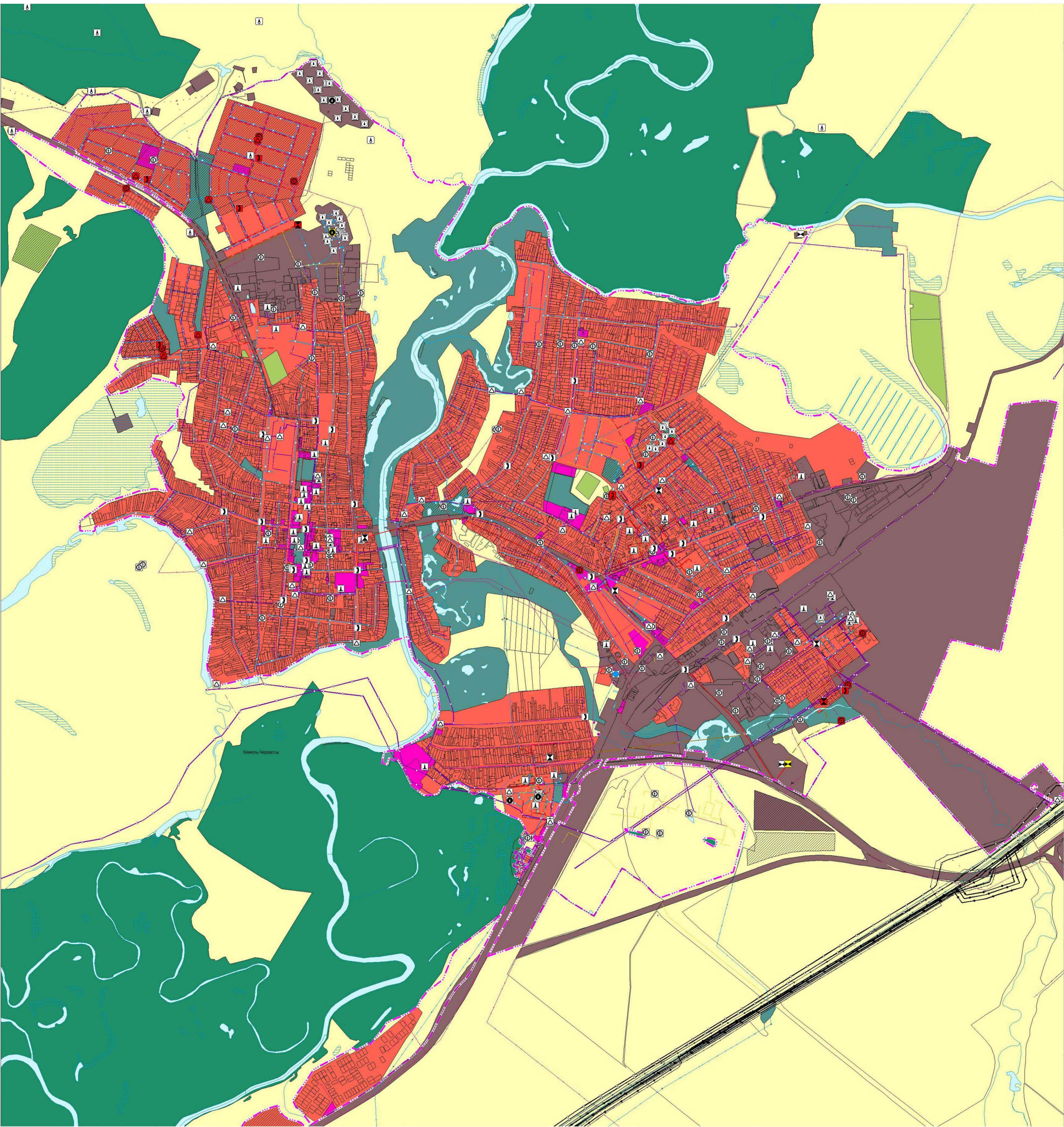
Карта планируемого размещения объектов инженерной инфраструктуры местного значения с. Кинель-Черкассы муниципального района Кинель-Черкасский Самарской области
