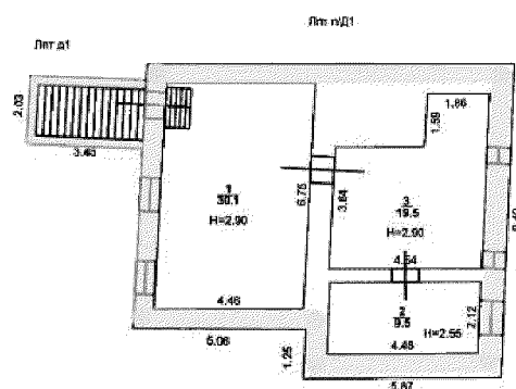
план подвала
