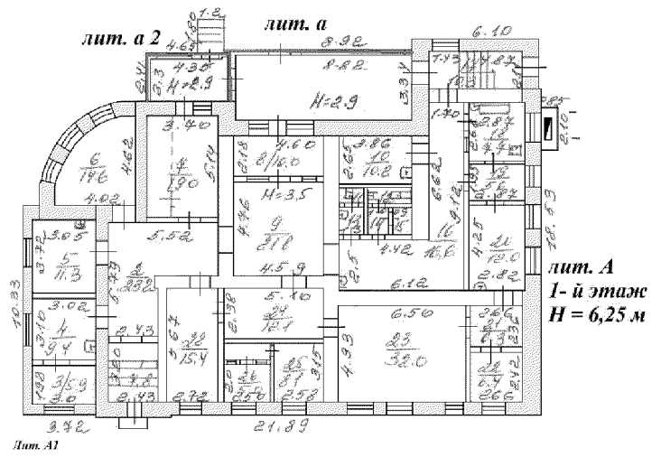
план первого этажа условные обозначения:
