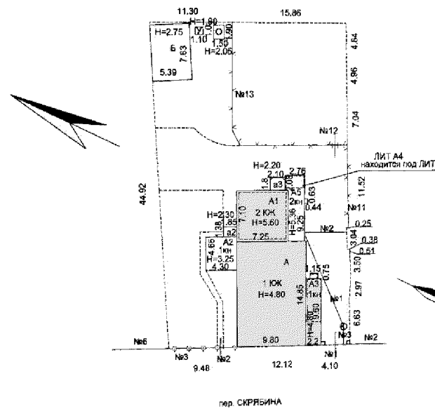
ситуационный план земельного участка, источник: техническое дело МУП ЦТИ г. Новочеркаска № 1589, 2014 г.
