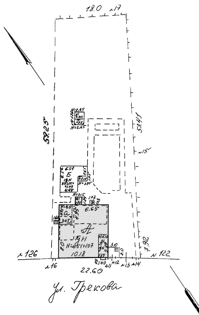
план домовладения объекта культурного наследия
