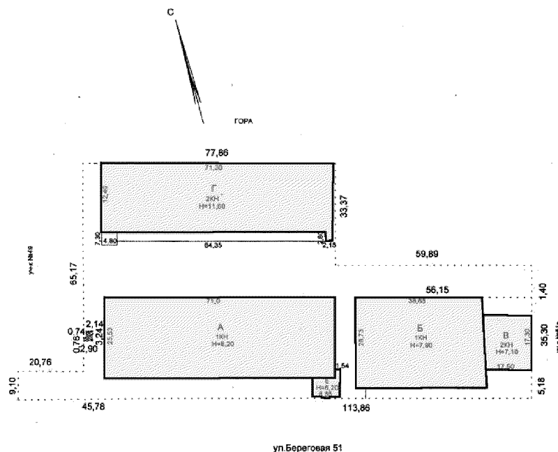
ситуационный план земельного участка по адресу: ул. Береговая, 51, литеры А, Е; ул. Береговая, 51, литеры Б, В; ул. Береговая, 51, литер Г
