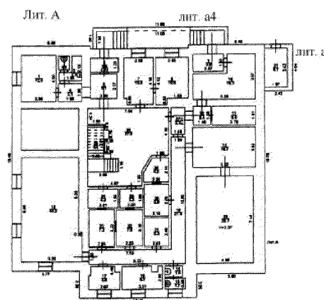
план цокольного этажа объекта культурного наследия, литеры п/А, А, а;
