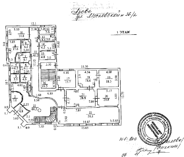
план 1-го этажа объекта культурного наследия;
