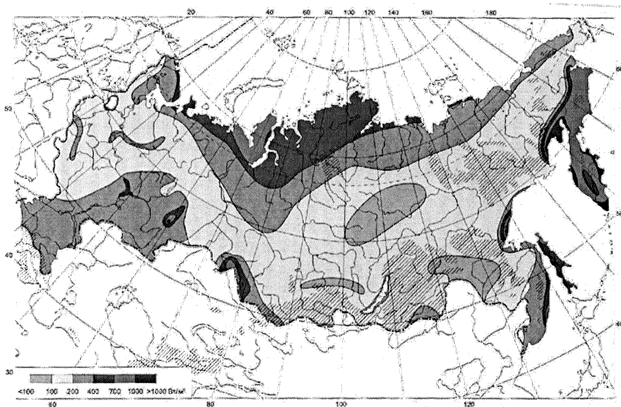
Рисунок 18 – Распределение удельного ветропотенциала (Вт/м 2 ) на высоте 100 м на территории Российской Федерации
