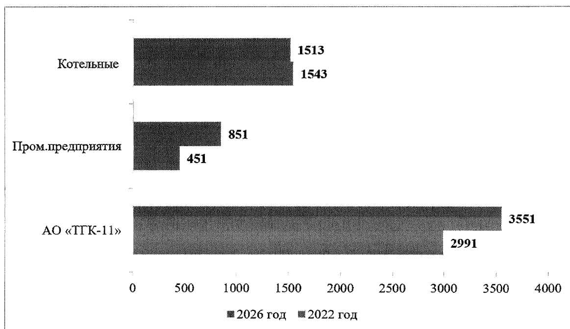
Рисунок 27 – Сравнительная диаграмма прогнозируемого расхода топлива по ТЭС и котельным за 2022 и 2026 годы (региональный вариант), т.у.т.
