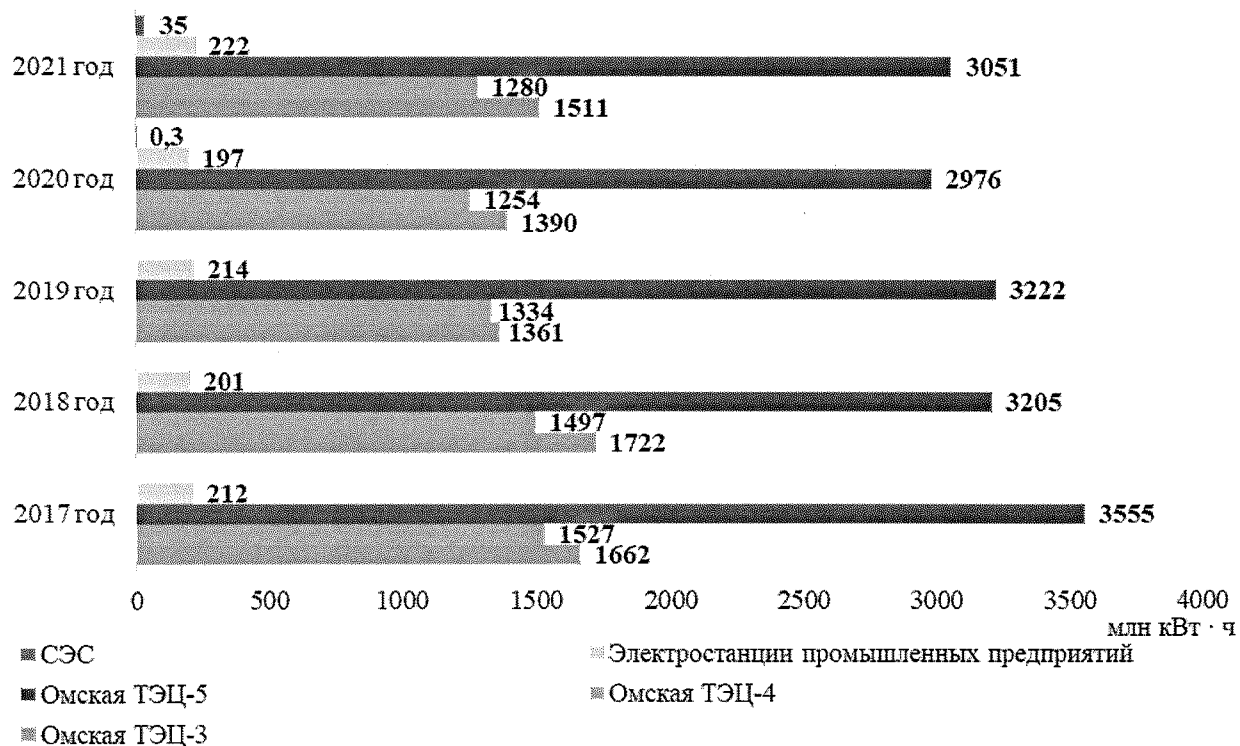
Рисунок 7 – Структура выработки электрической энергии на электростанциях ЭС Омской области за 2017 – 2021 годы
