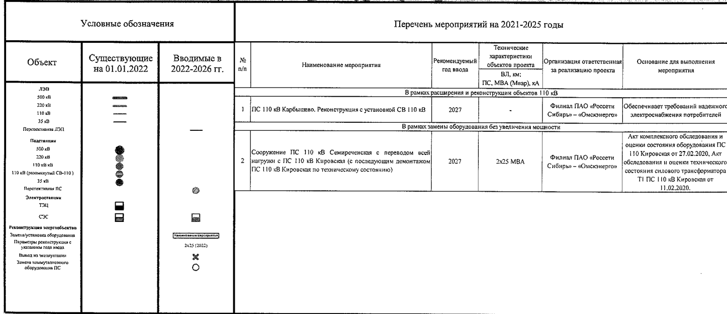
Рисунок 1.2 - Карта-схема электрических сетей 110 кВ и выше г. Омск на 2022-2026 годы. Базовый вариант развития
