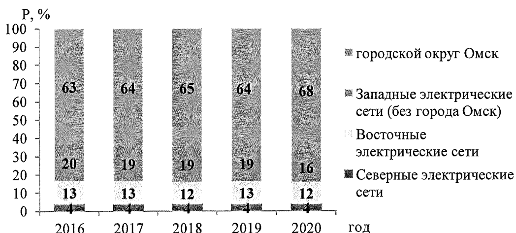
Рисунок 5 – Структура потребления мощности энергорайонов ЭС Омской области за отчетный период
