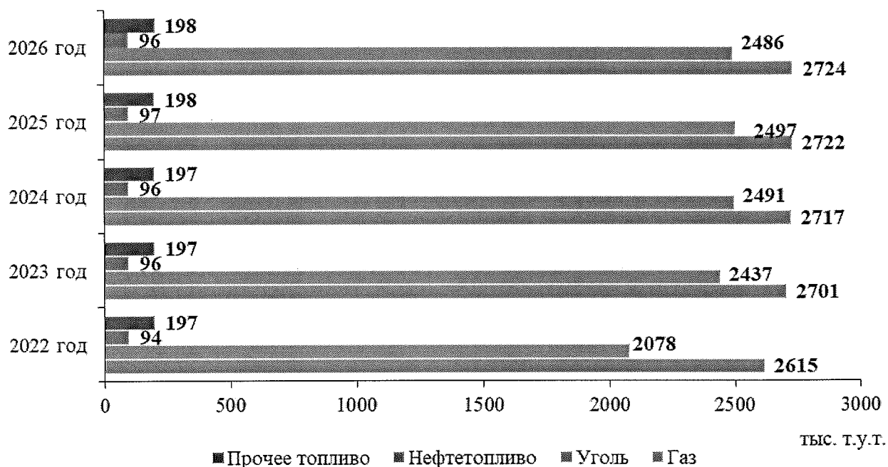
Рисунок 24 – Прогноз потребности в топливе ТЭС и котельных Омской области для базового уровня электропотребления, тыс. т у.т.
