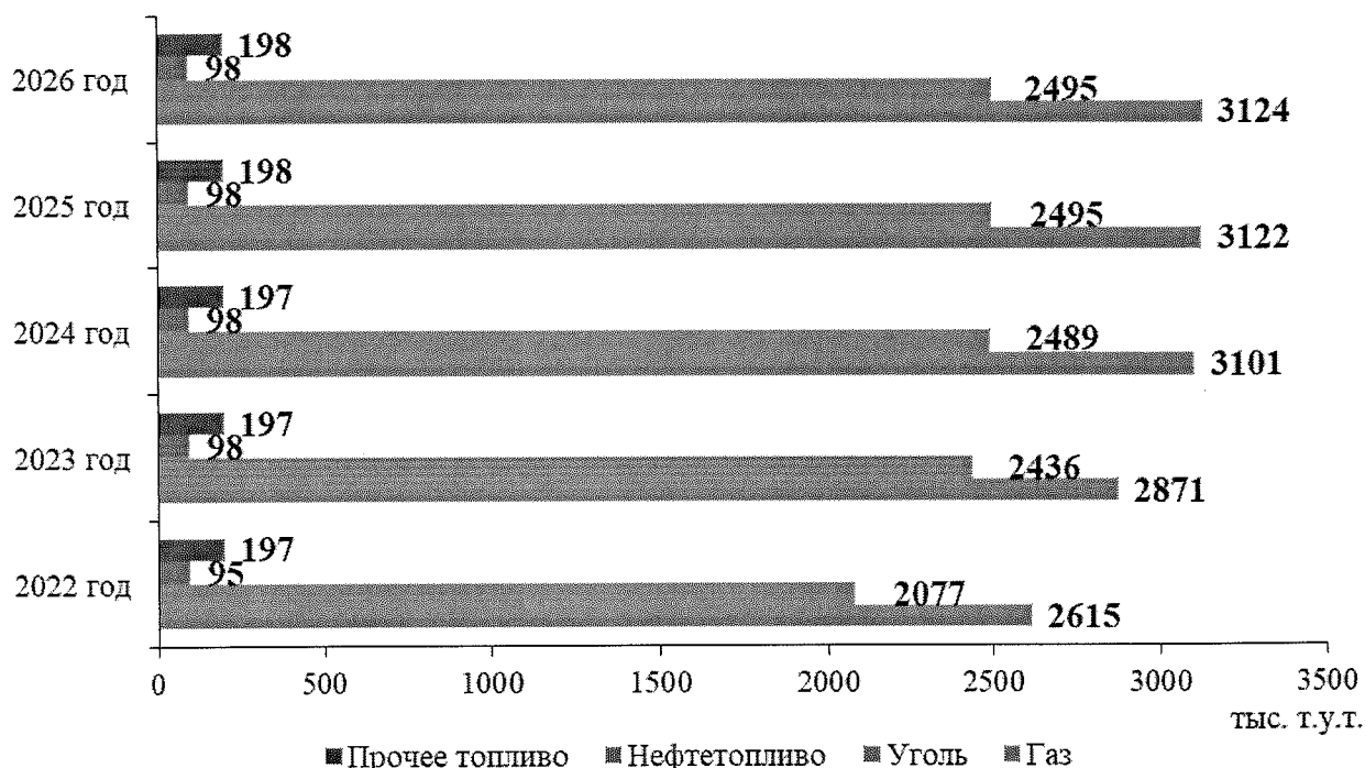
Рисунок 25 – Прогноз потребности в топливе ТЭС и котельных Омской области для регионального уровня электропотребления, тыс. т у.т.
