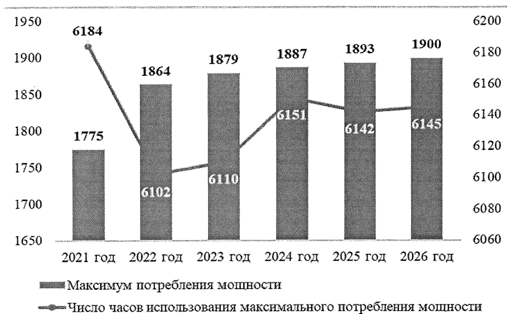
Рисунок 16 – Динамика изменения максимального потребления электрической мощности и числа часов его использования для базового варианта электропотребления
