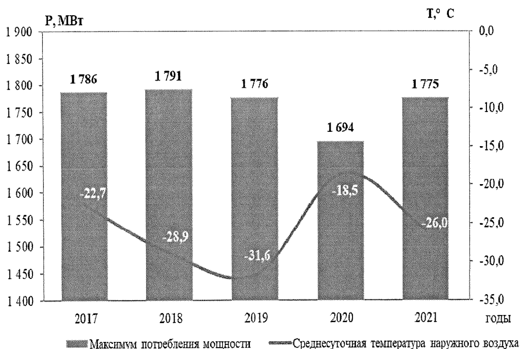
Рисунок 4 – Динамика изменения максимального потребления электрической мощности ЭС Омской области и температуры наружного воздуха за 2017 – 2021 годы
