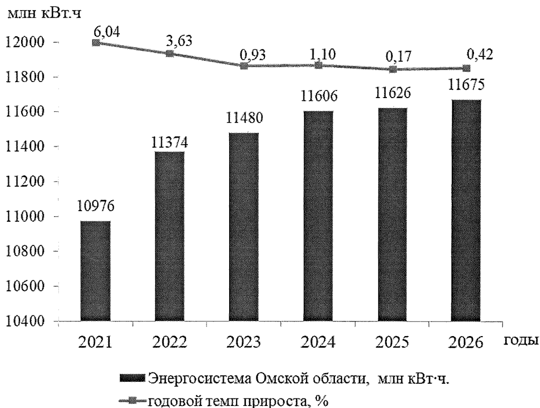
Рисунок 14 – Прогноз спроса на электрическую энергию по ЭС Омской области за период 2022 – 2026 годов. Базовый вариант
