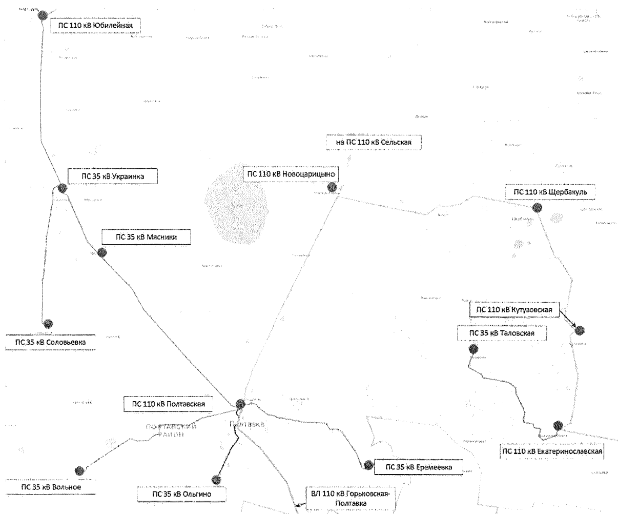
Рисунок 23 – Карта-схема электрических сетей напряжением 35 – 110 кВ энергорайона размещения ПС 110 кВ Полтавская
