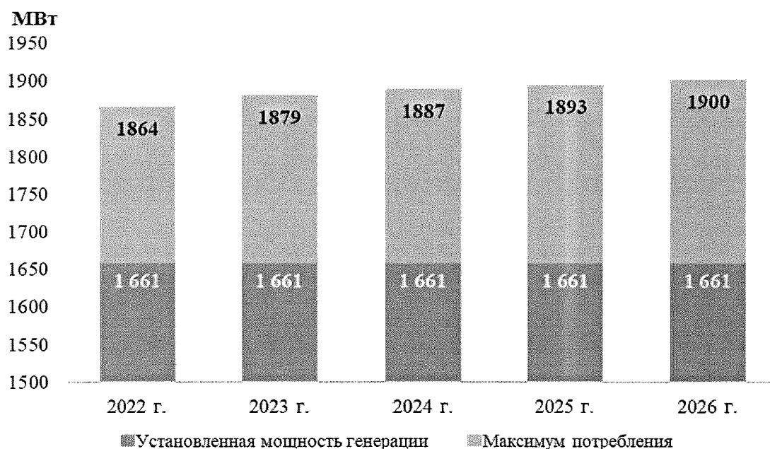
Рисунок 21 – Перспективный баланс мощности ЭС Омской области на 2022 – 2026 годы по базовому варианту развития
