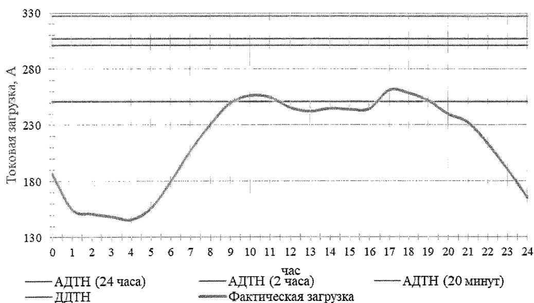
Рисунок 13 – Суточный график загрузки ПС 110 кВ Энтузиастов с учетом реализации ТУ на ТП
