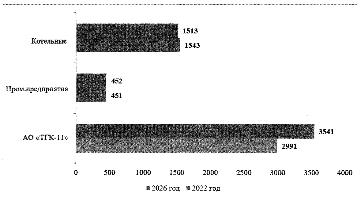
Рисунок 26 – Сравнительная диаграмма прогнозируемого расхода топлива по ТЭС и котельным за 2022 и 2026 годы (базовый вариант), т.у.т.
