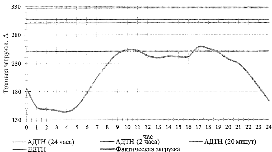
Рисунок 12 – Суточный график загрузки ПС 110 кВ Энтузиастов
