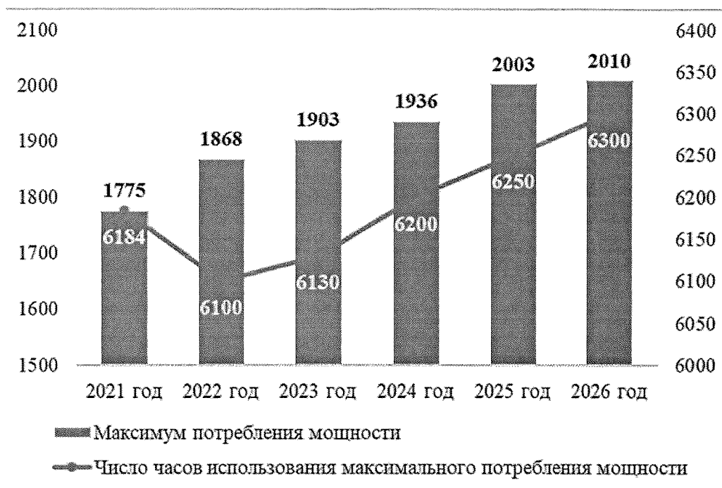
Рисунок 17 – Перспективные режимы электропотребления ЭС Омской области для дополнительного варианта электропотребления
