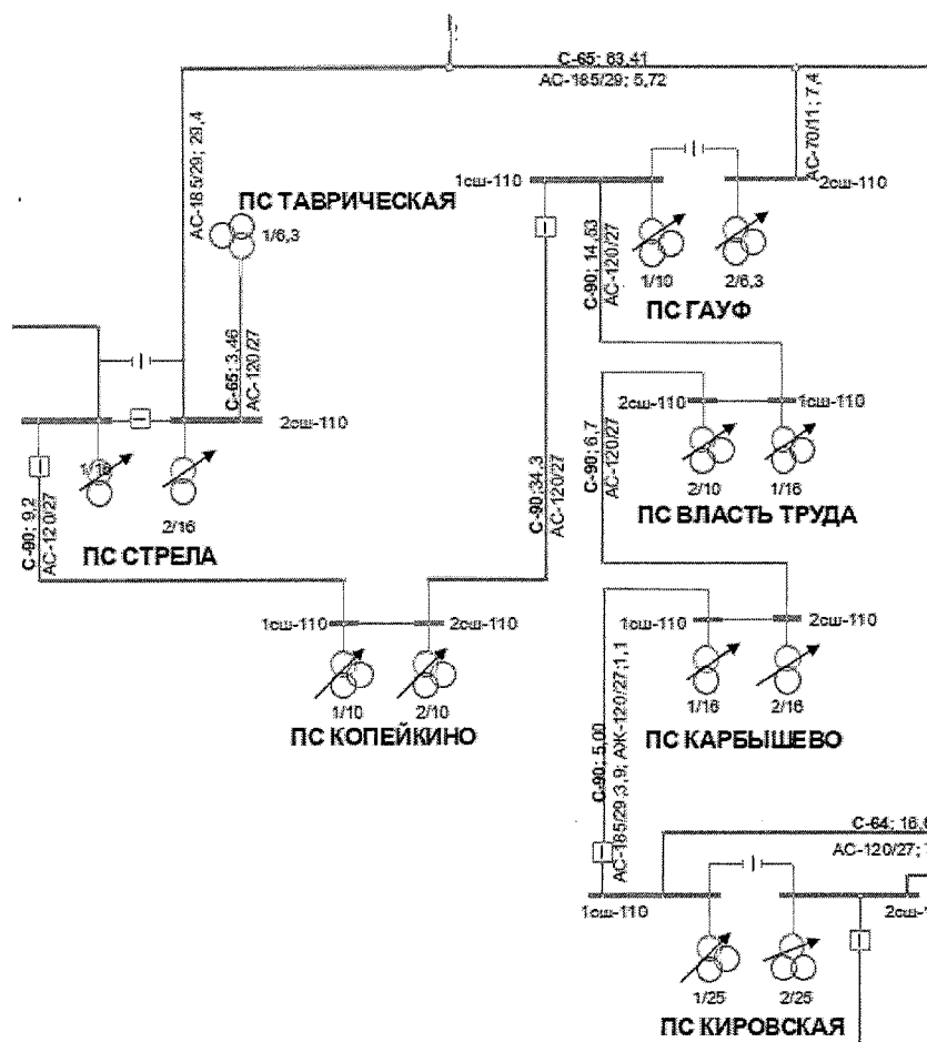
Рисунок 11 – Схема сети 110 кВ в районе ПС 110 кВ Карбышево
