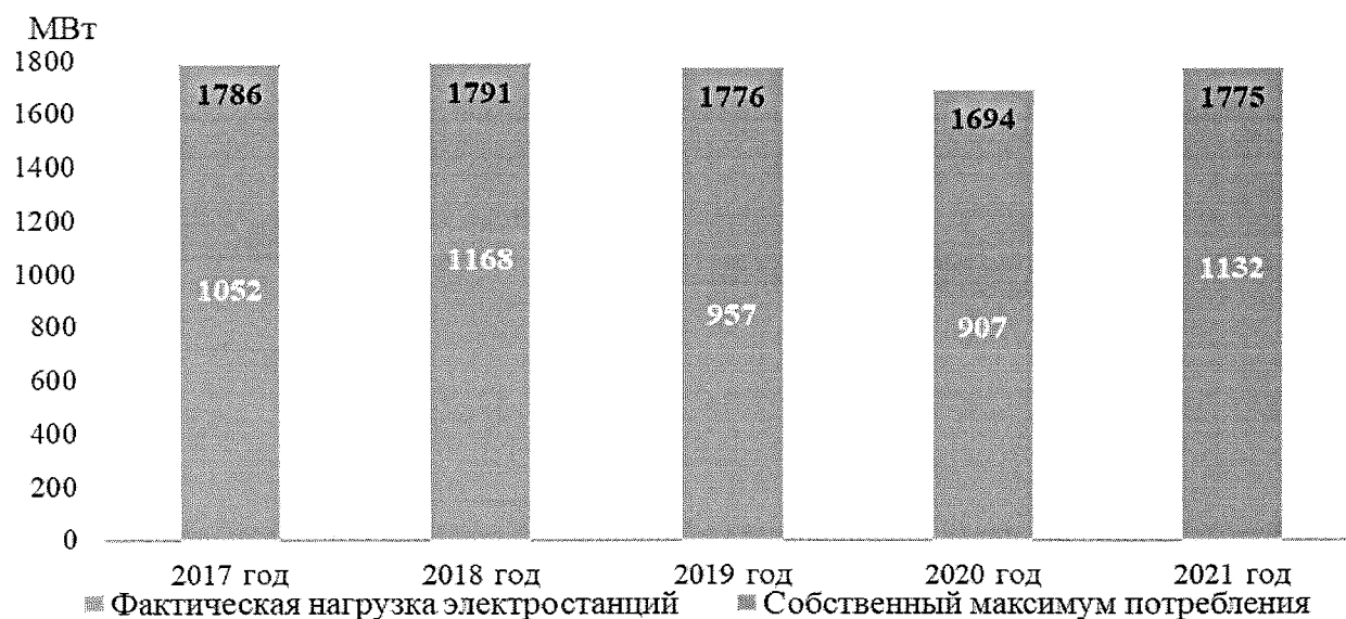
Рисунок 9 – Баланс мощности ЭС Омской области на час прохождения максимума потребления ЭС за 2017 – 2021 годы
