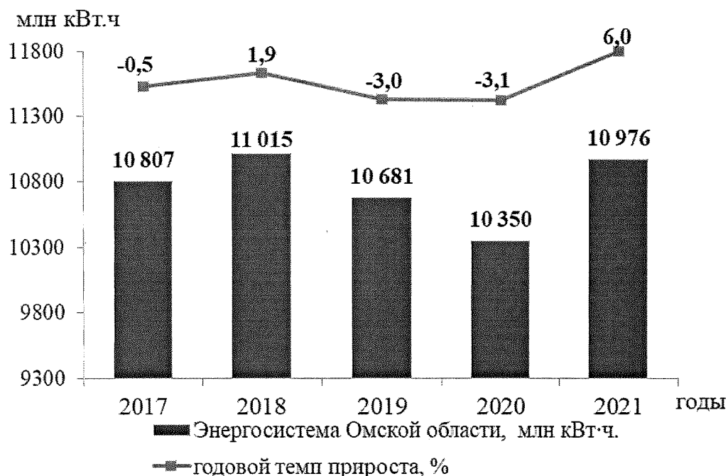
Рисунок 2 – Динамика потребления электроэнергии в Омской области за последние 5 лет
