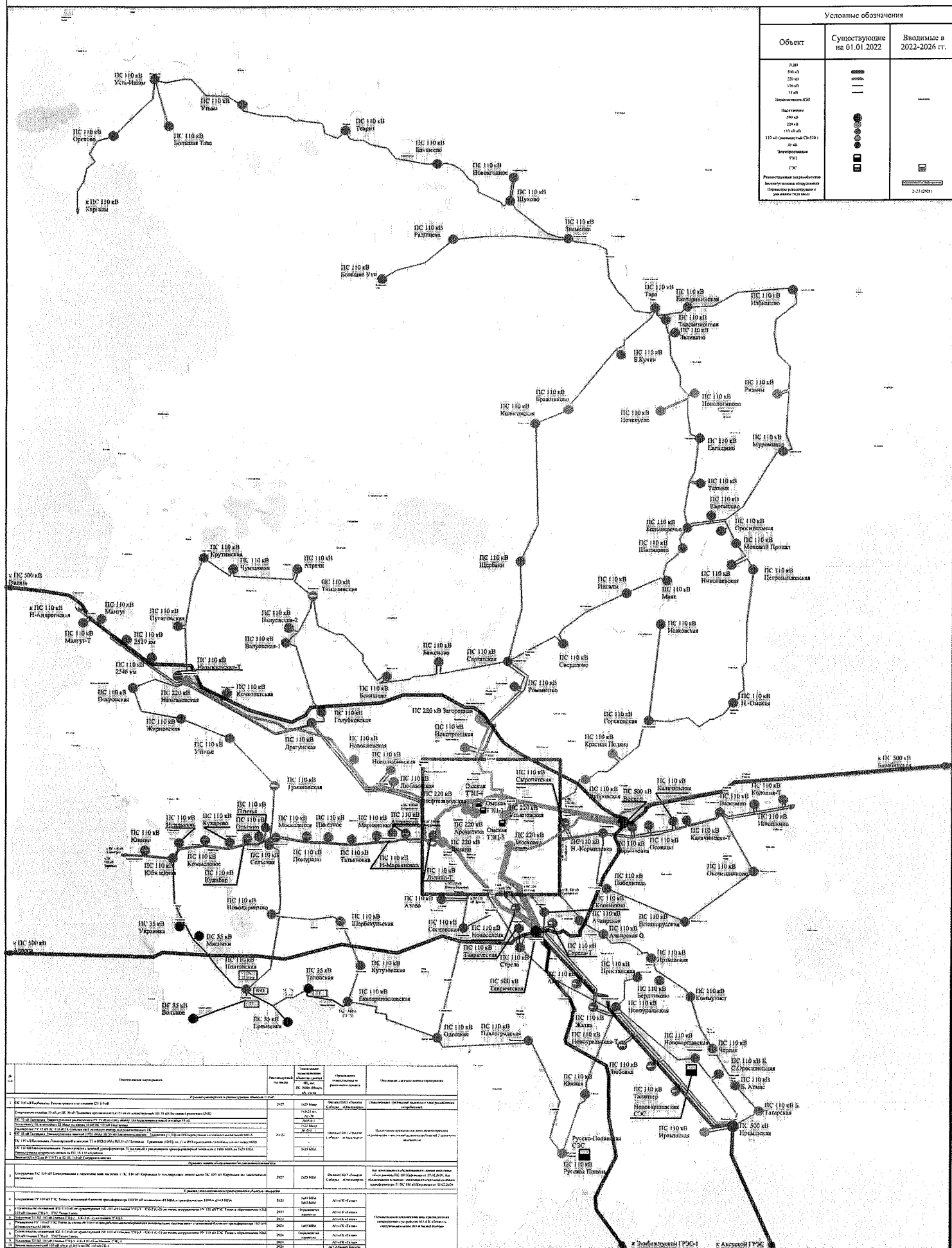
Рисунок 1.3 - Карта схема электрических сетей 110 кВ и выше Омской области на период 2022-2026 годы. Дополнительный вариант развития
