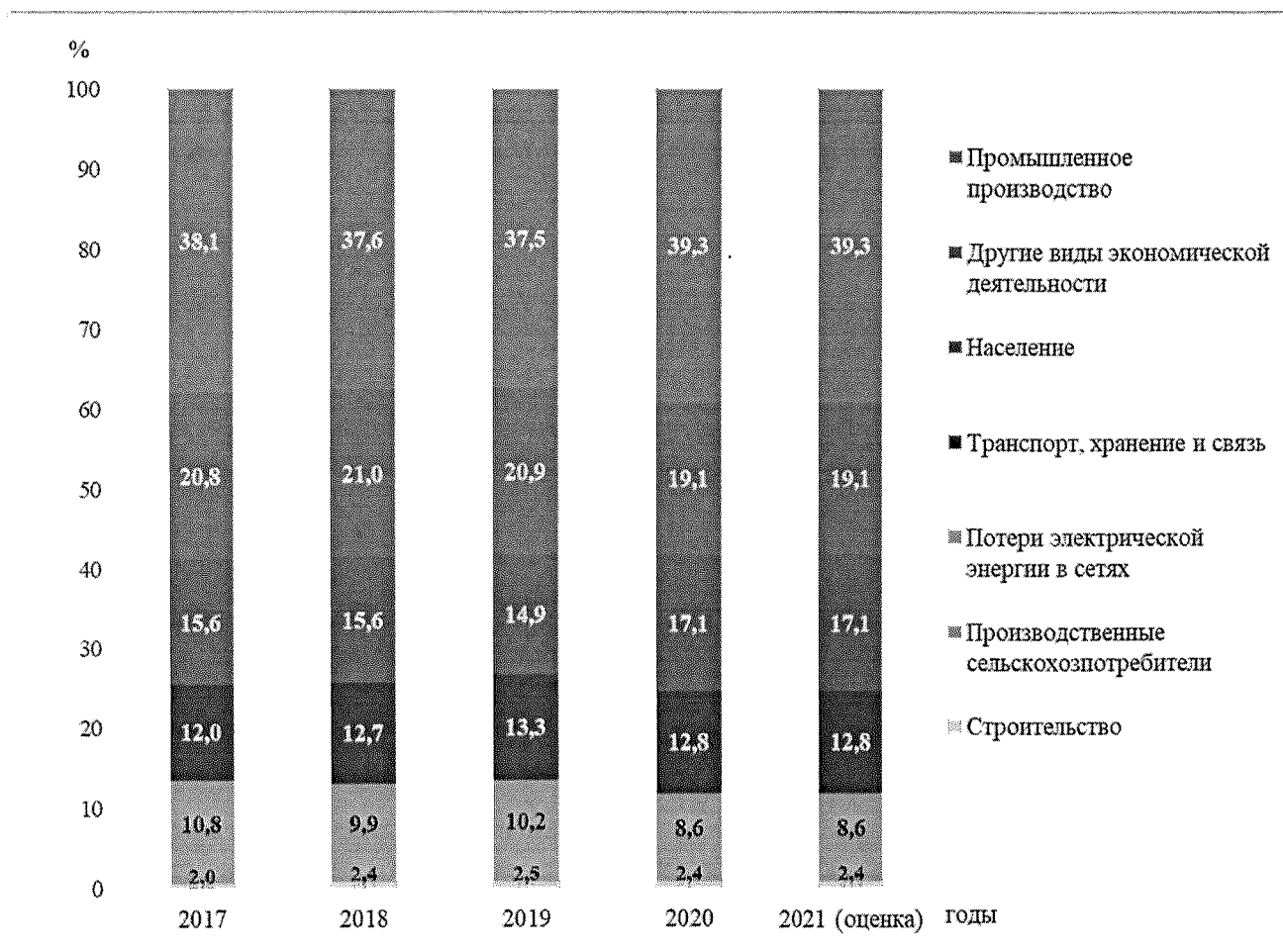
Рисунок 3 – Структура электропотребления по основным группам потребителей Омской области за период 2017 – 2021 годов
