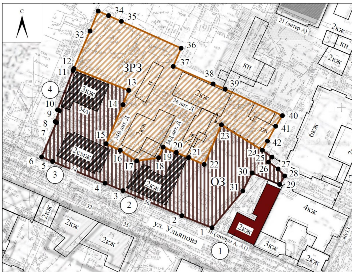
Схема координат
