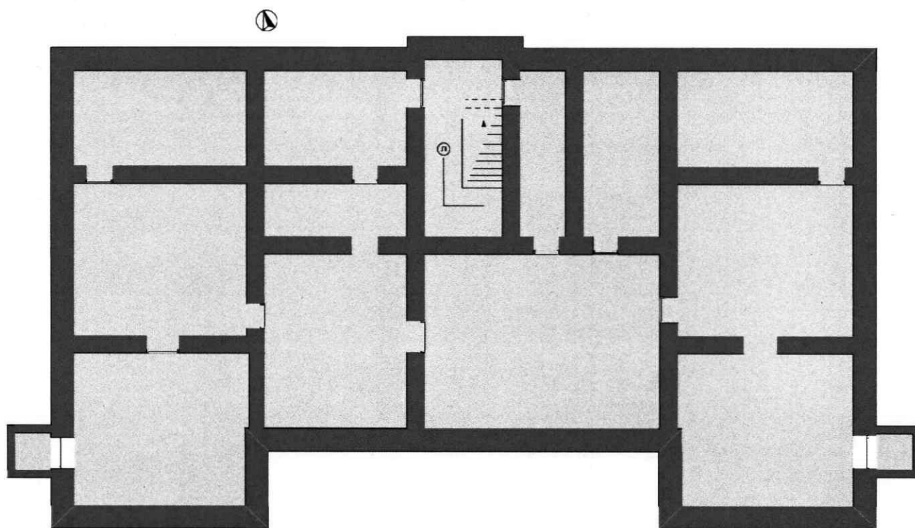
План подвала
