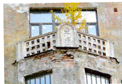
Ограждение балкона (крайний правый эркер, лицевой фасад)
