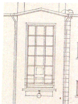
Фрагмент уличного Ю-З фасада. Проект 1931 г.
