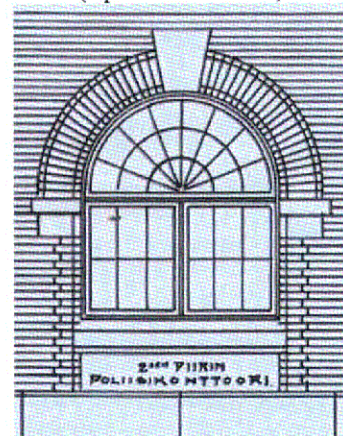
Рисунок расстекловки оконных проемов. Лицевой фасад (проект 1909 г.)
