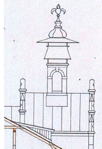
Башнеобразная надстройка. Вид сбоку. Проект 1909 г.
