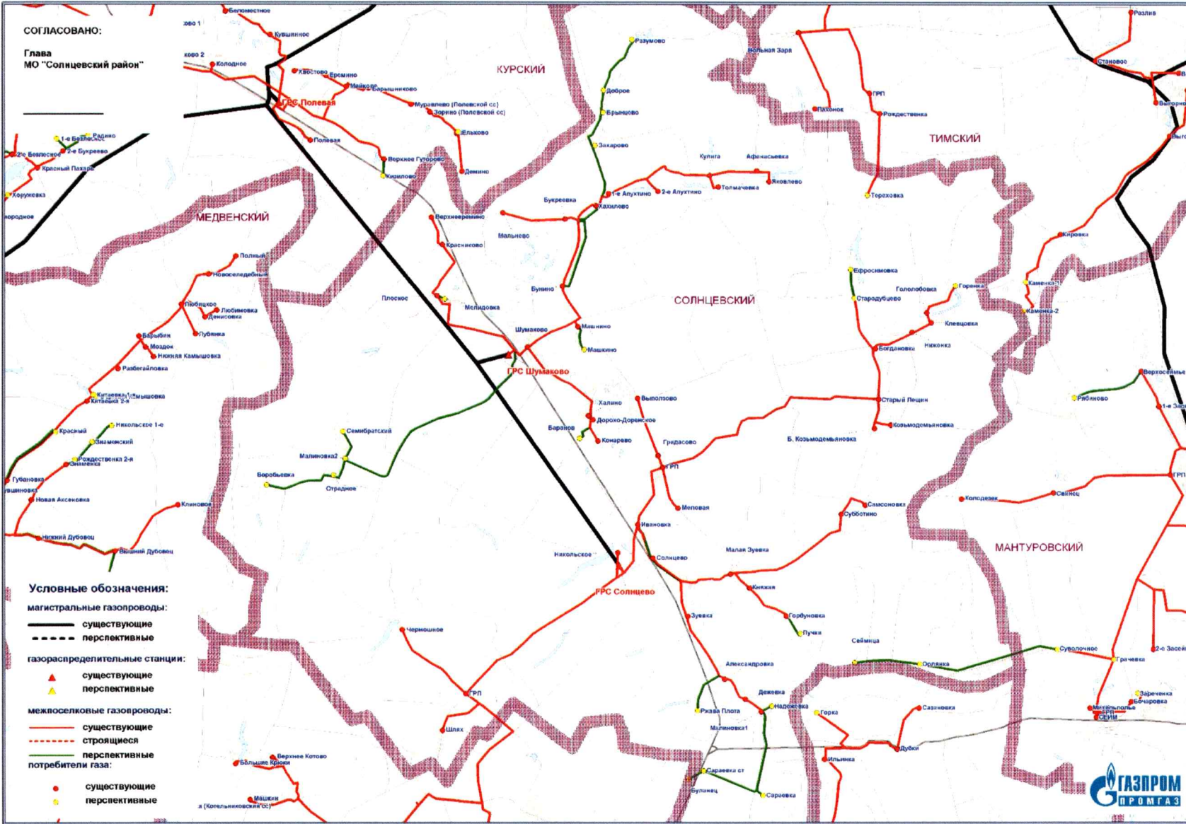
Схема газоснабжения и газификации Солнцевского района Курской области
