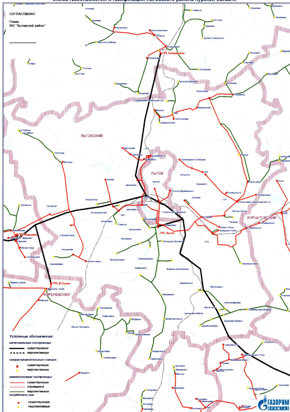
Схема газоснабжения и газификации Льговского района Курской области
