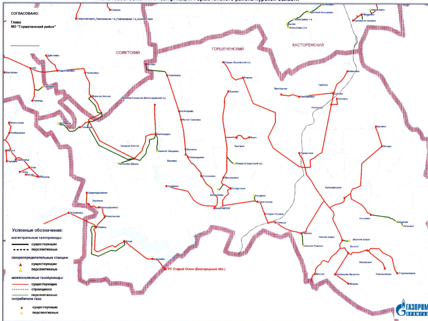
Схема газоснабжения и газификации Горшеченского района Курской области
