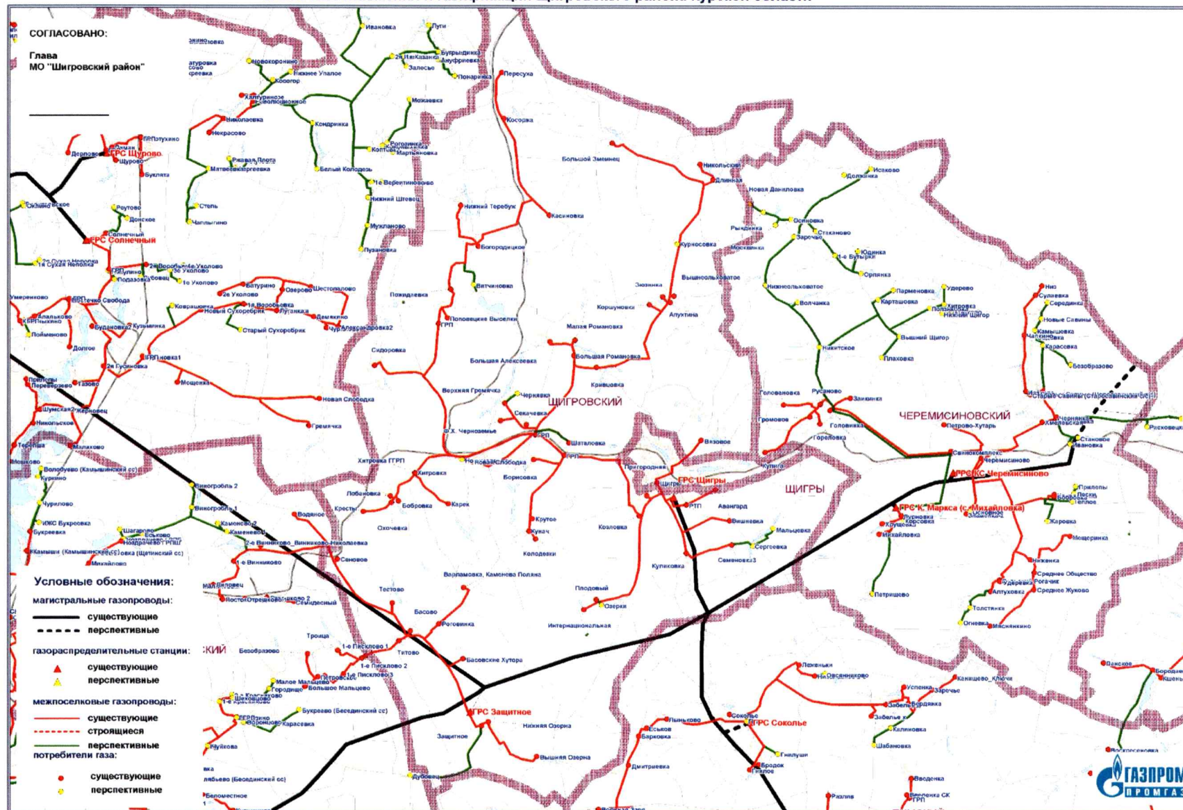
Схема газоснабжения и газификации Щигровского района Курской области
