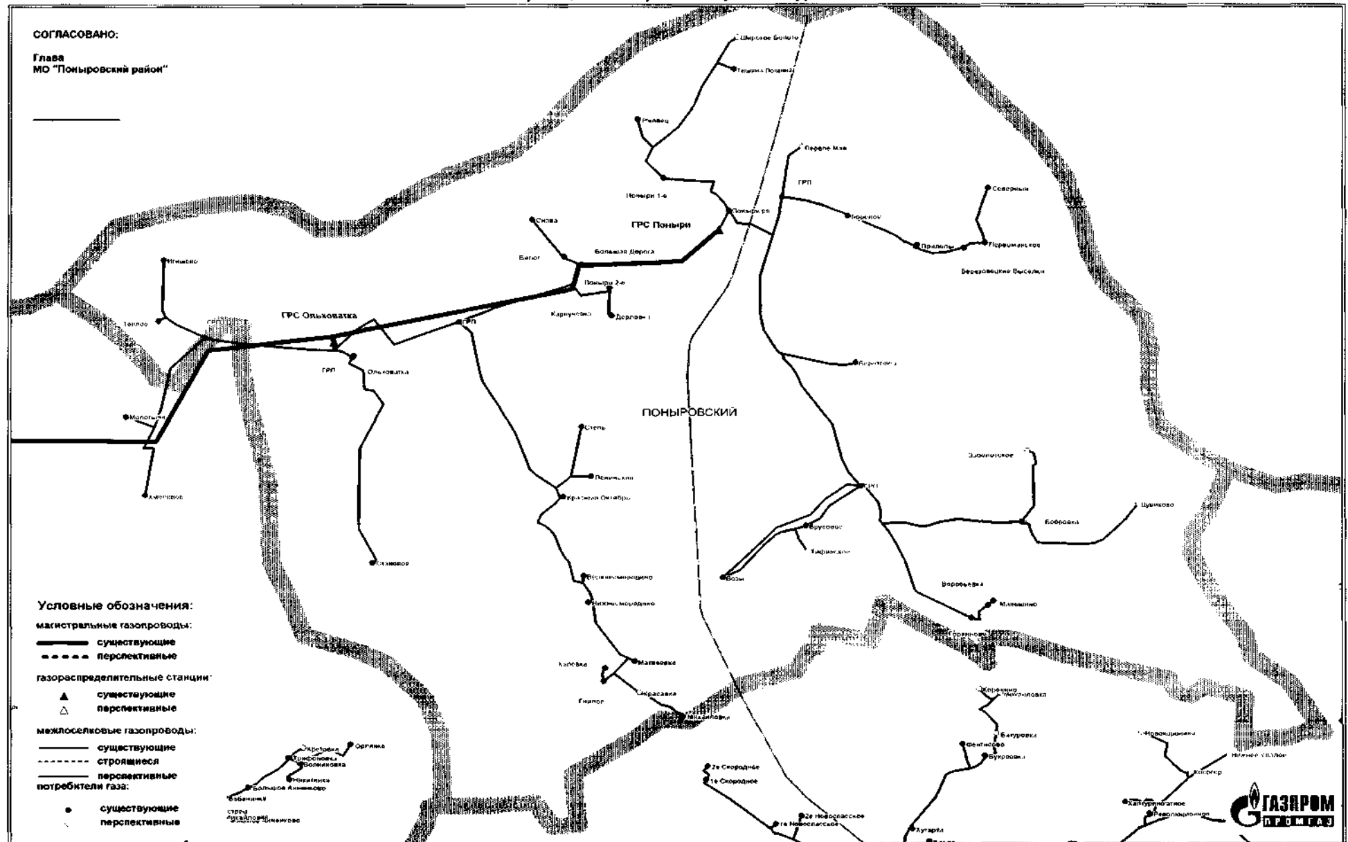
Схема газоснабжения и газификации Поныровского района Курской области
