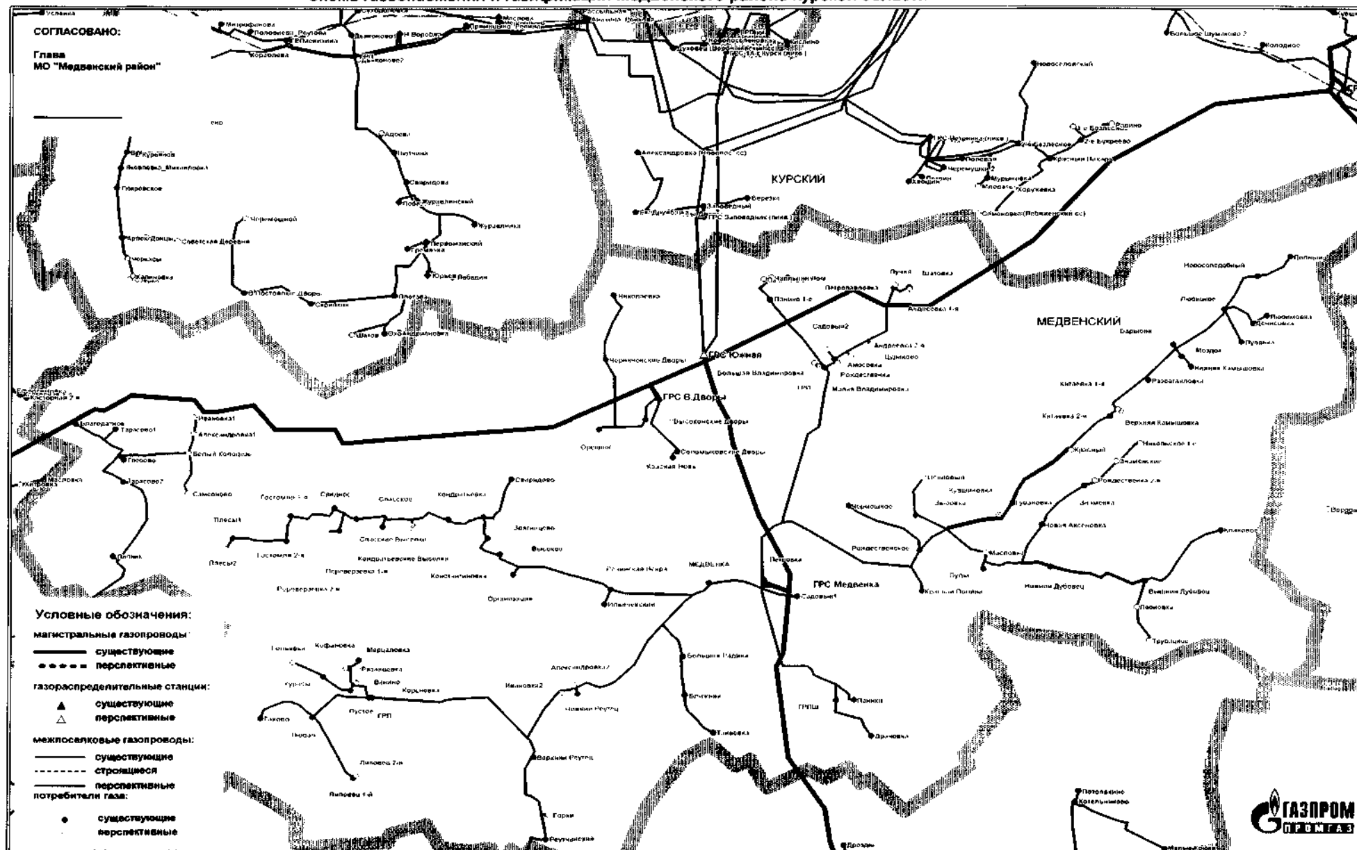
Схема газоснабжения и газификации Медвенского района Курской области
