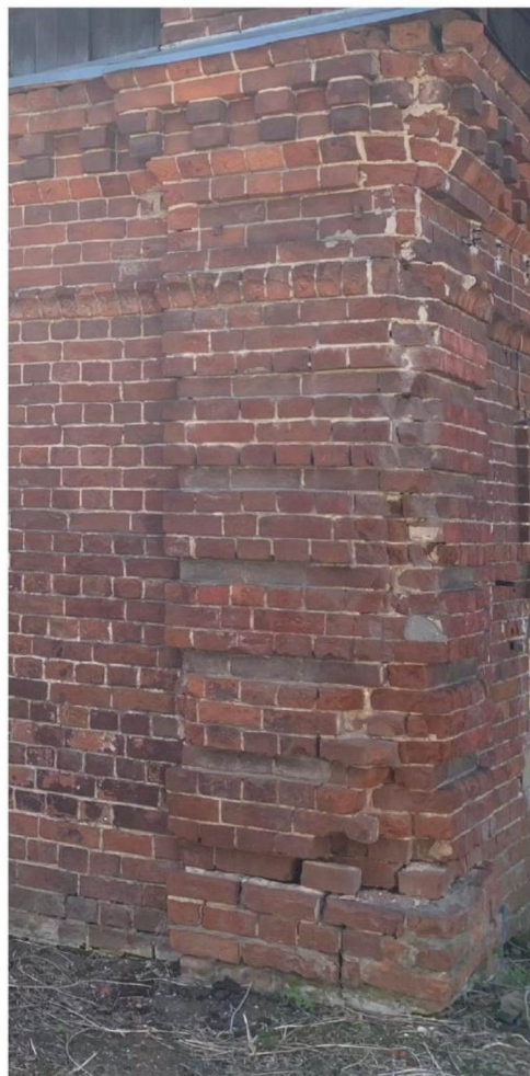
Вид рустованной лопатки с выносным венчающим карнизом.
