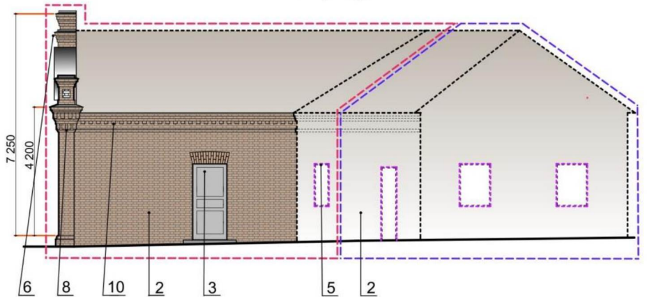
Южный фасад.
