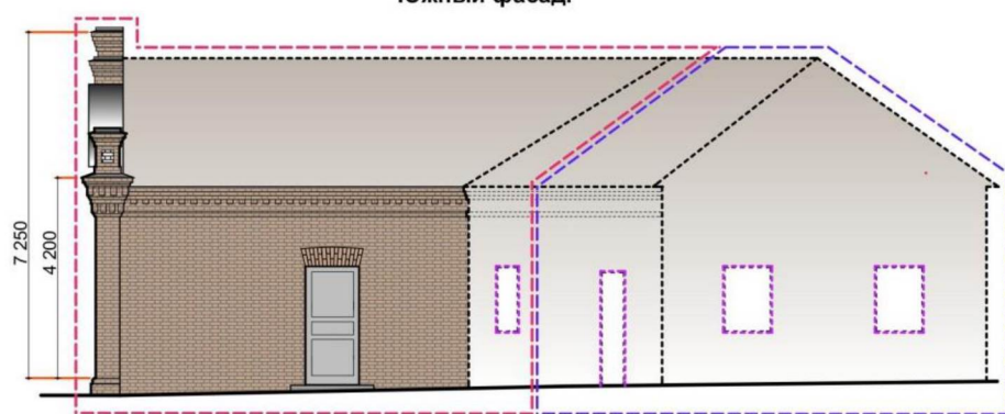
Южный фасад.
