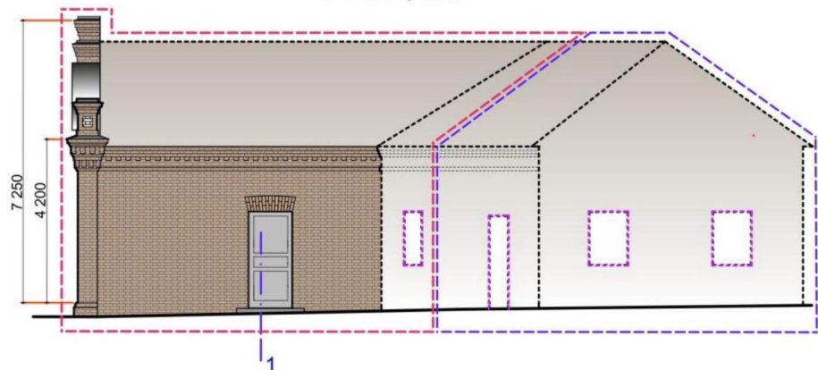
Южный фасад.
