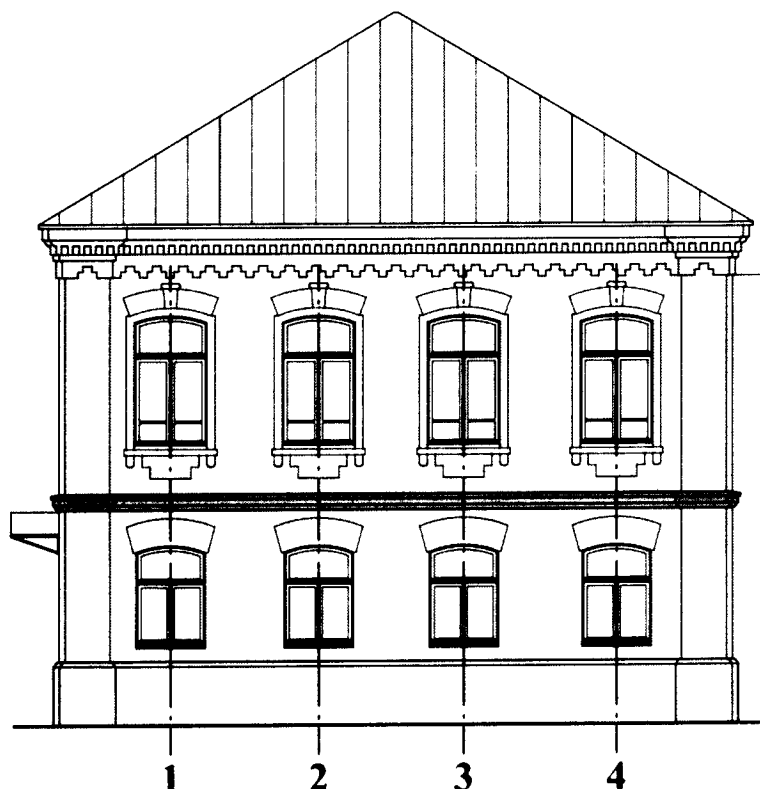
Освое членение фасадов Северо-западный фасад
