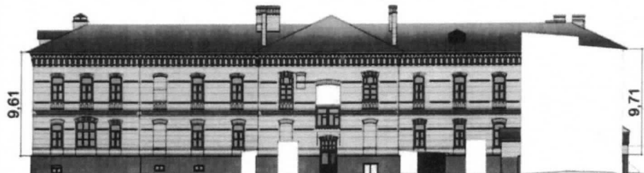
Северо-восточный фасад
