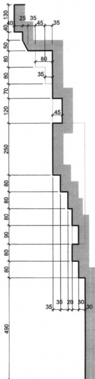
Профиль каменного подоконника. М 1:2
