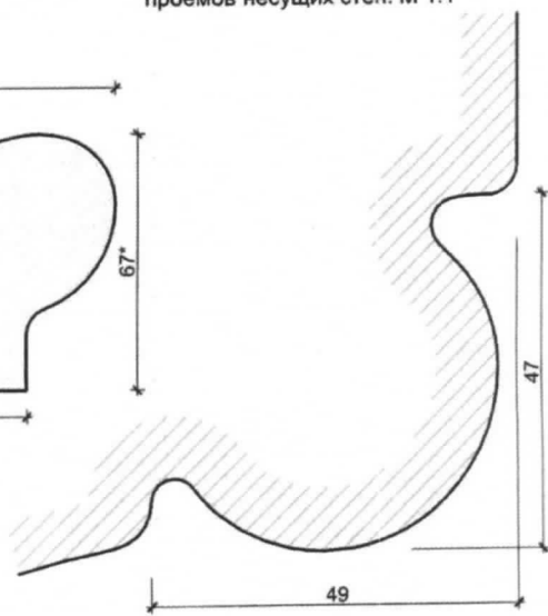
Деталь. Профиль филенок в толще проемов несущих стен. М 1:1
