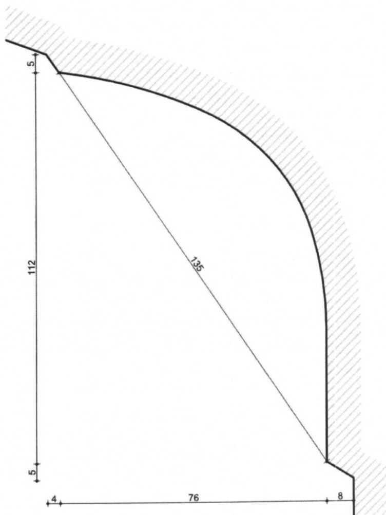
Потолочная падуга. М 1:1
