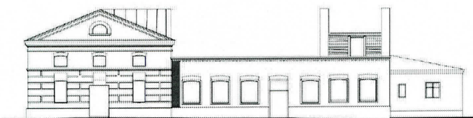
Восточный фасад
