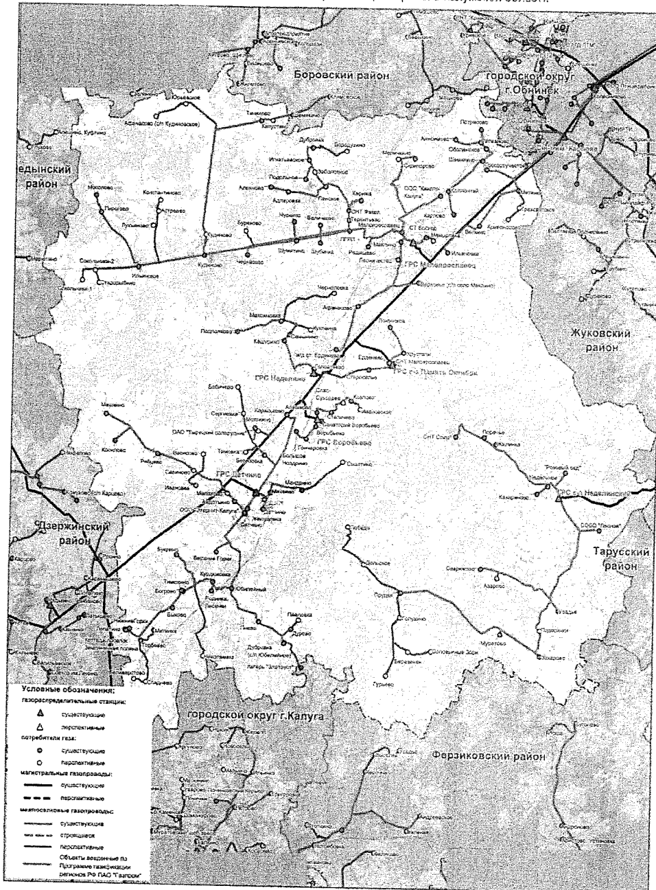
Схема газоснабжения и газификации Малоарского района Калужской области
