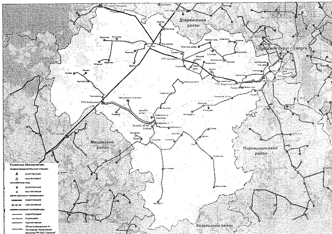
Схема газоснабжения и газификации Бабьинского района Калужской области
