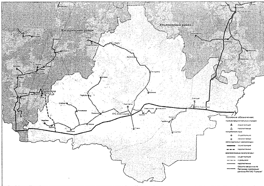
Схема газоснабжения и газификации Южнодновского района Калужской области
