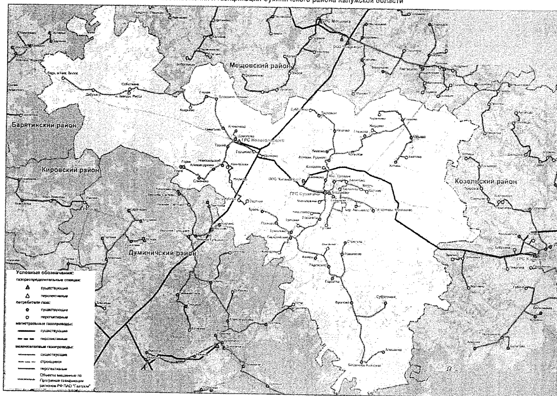
Схема газоснабжения и газификации Сухиничского района Калужской области
