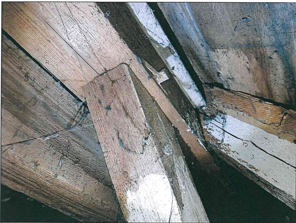
Фото 75. Чердак. Конструкции стропильной системы крыши.
