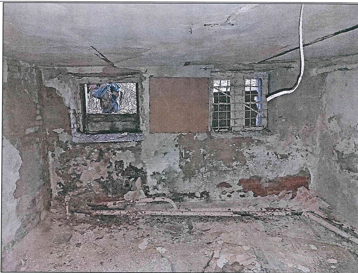
Фото 46. Подвал. Конструкции стен, перекрытий. Конструкции оконных проемов.
