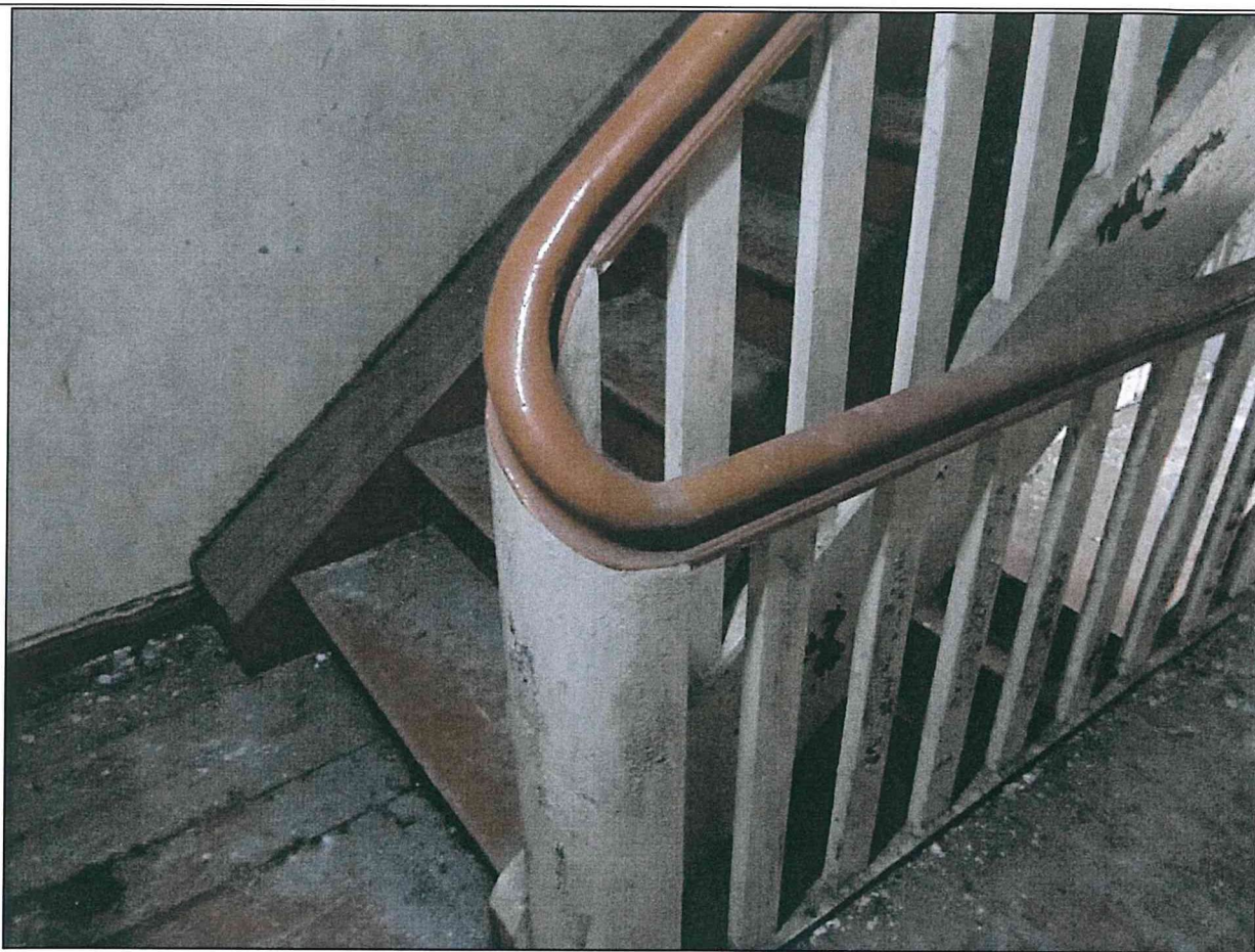
Фото 70. Третий этаж – мансарда. Конструкции межэтажной лестницы, межэтажная площадка.
