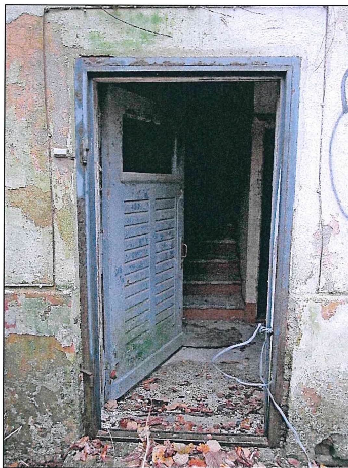
Фото 49. Первый этаж. Фасад № 3 – дворовый вход. Конструкции дверного заполнения.
