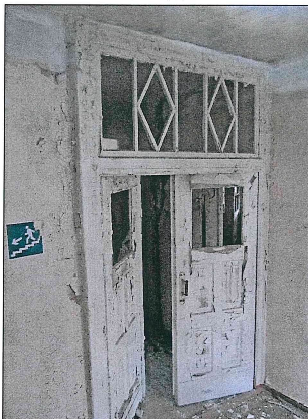
Фото 60. Второй этаж. Конструкции стен, перекрытий. Дверной проем входа во внутренние помещения второго этажа. Конструкция дверного заполнения.
