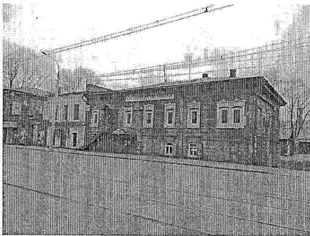
Фото 1. Главный фасад по улице Тимирязева дома под лит. а.
