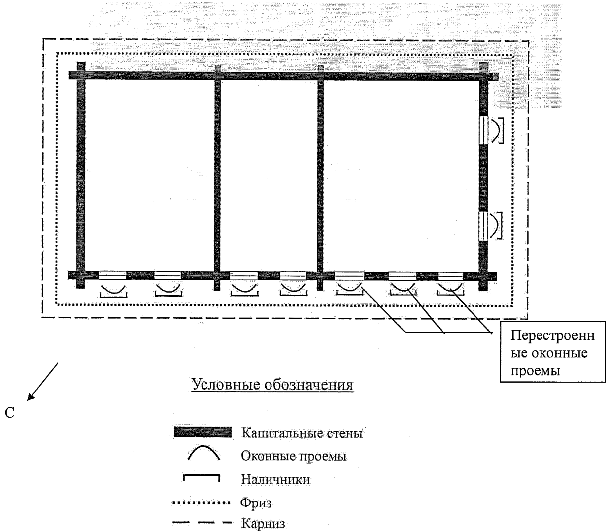
Схема обозначения предмета охраны в уровне 1 этажа
