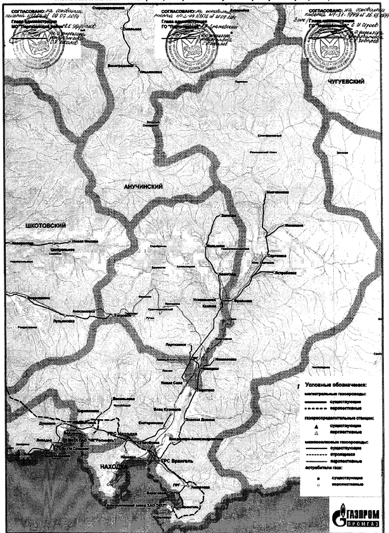
Схема газоснабжения и газификации Партизанского района Приморского края (2014г.)
